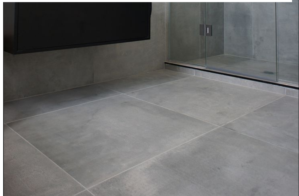
Dacite (Zerde Tile)
